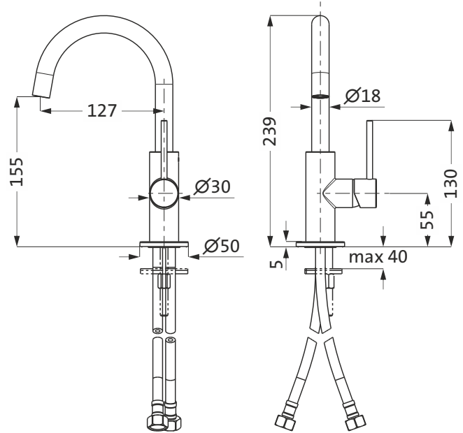
Lochbohrung 35mm
