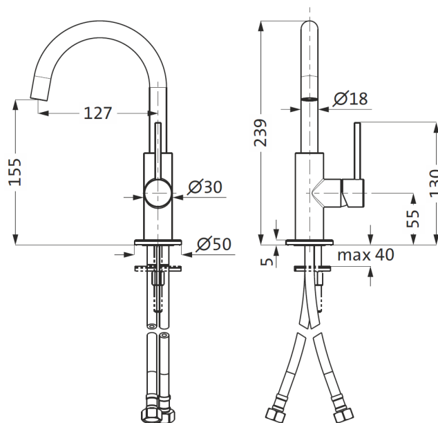
Lochbohrung 35mm
