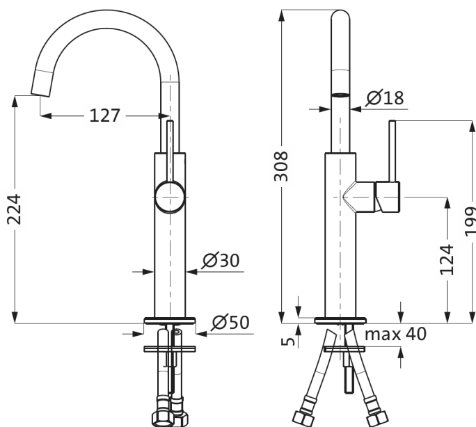
Lochbohrung 35mm
