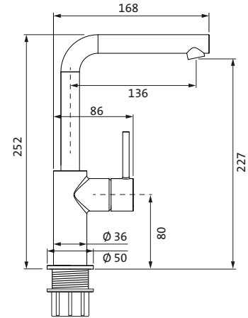
Lochbohrung \varnothing 35 mm hole diameter
